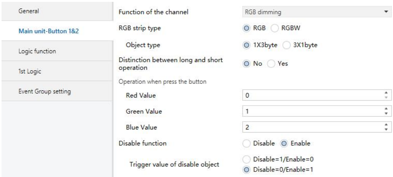
图 4.9 “Main unit-Button x: RGB dimming”参数设置界面（1）
