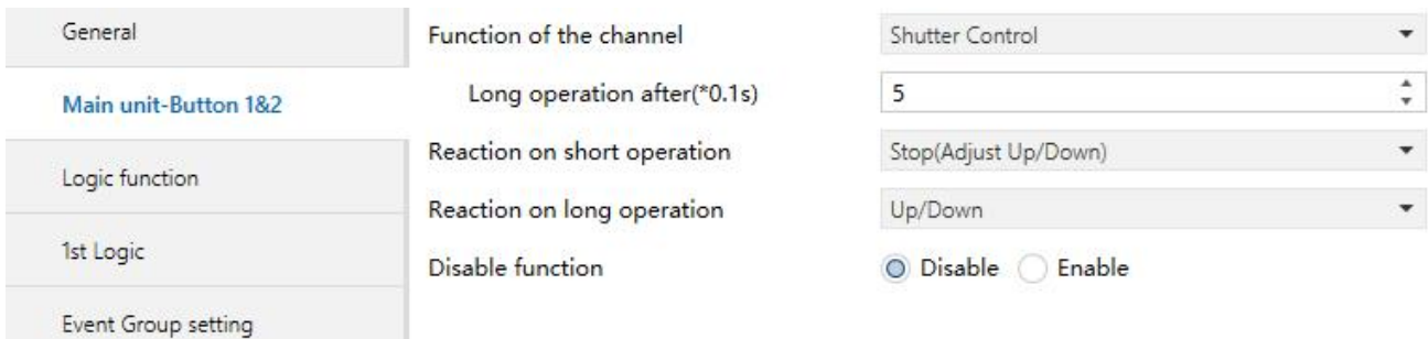
图 4.7 参数设置界面“Main unit-Button x: Shutter control”
