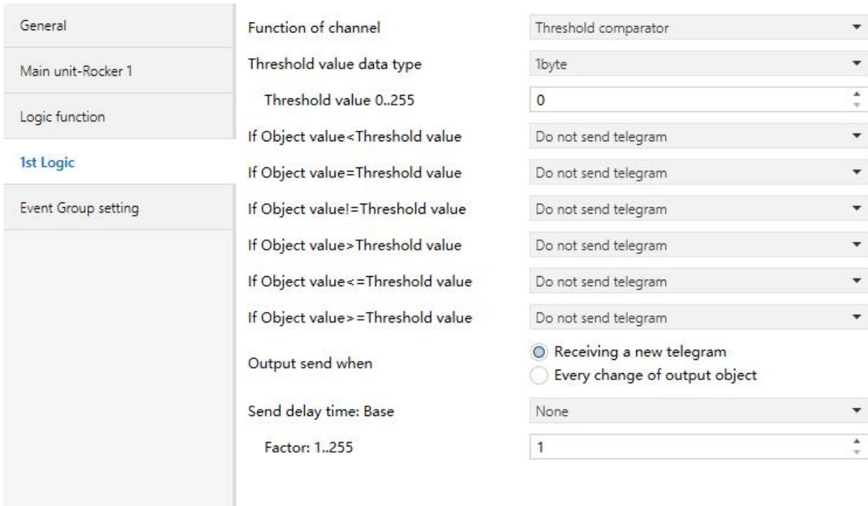
图 4.23 参数设置界面“Logic function -- Threshold comparator”
