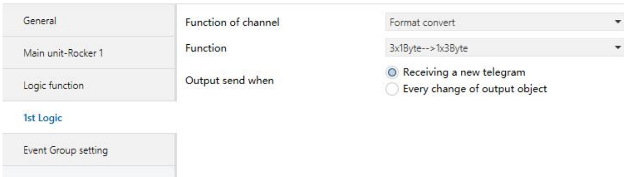
图 4.24 参数设置界面“Logic function -- Format convert”
