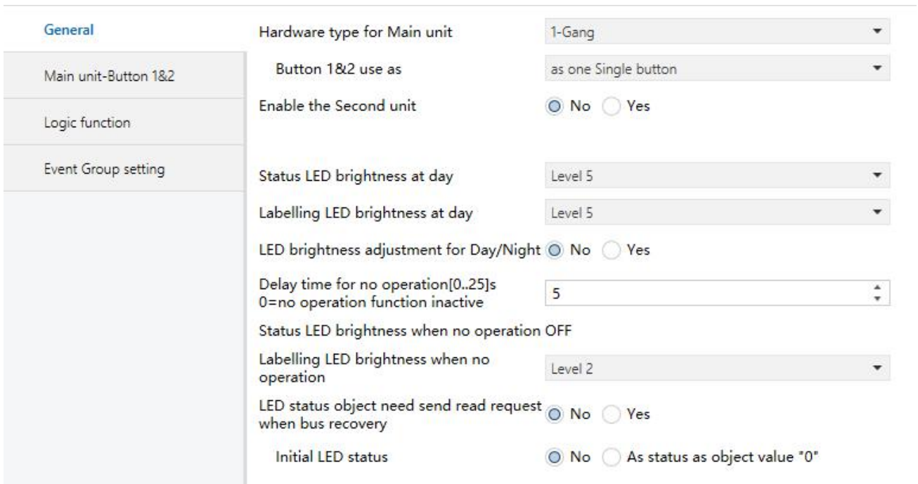
图 4.1 “General”参数设置界面
