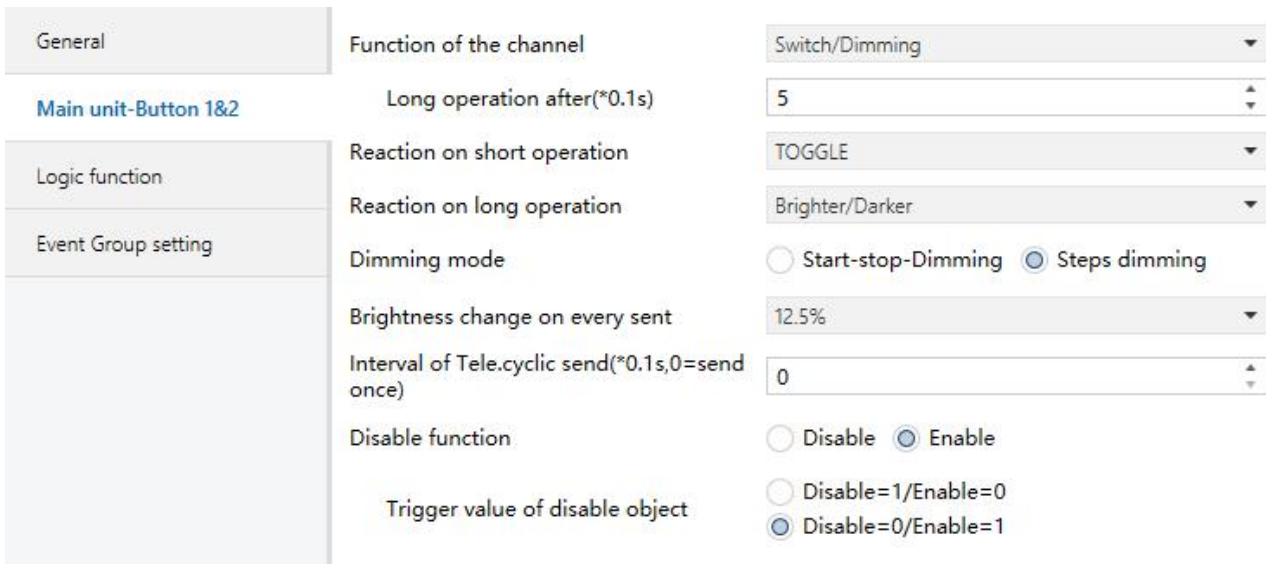
图 4.4 参数设置界面“Main unit-Button X:Switch/Dimming”
